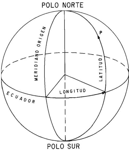
Esquema de las coordenadas geográficas básicas.
