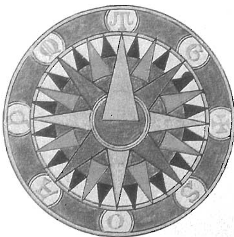
Rosa náutica procedente de la derrota de Elcano.
